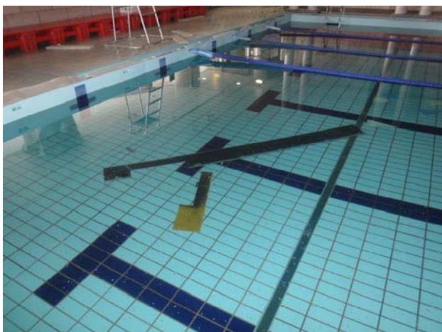
① プール天井落下
