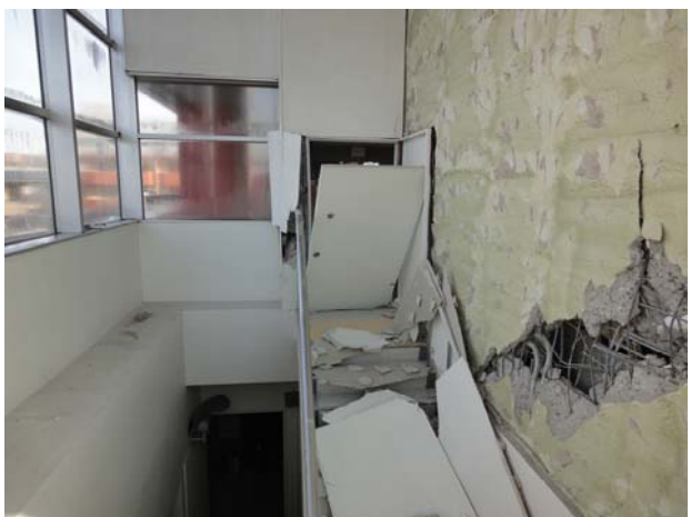
③ 壁崩落（男子更衣室側：2階から3階）
